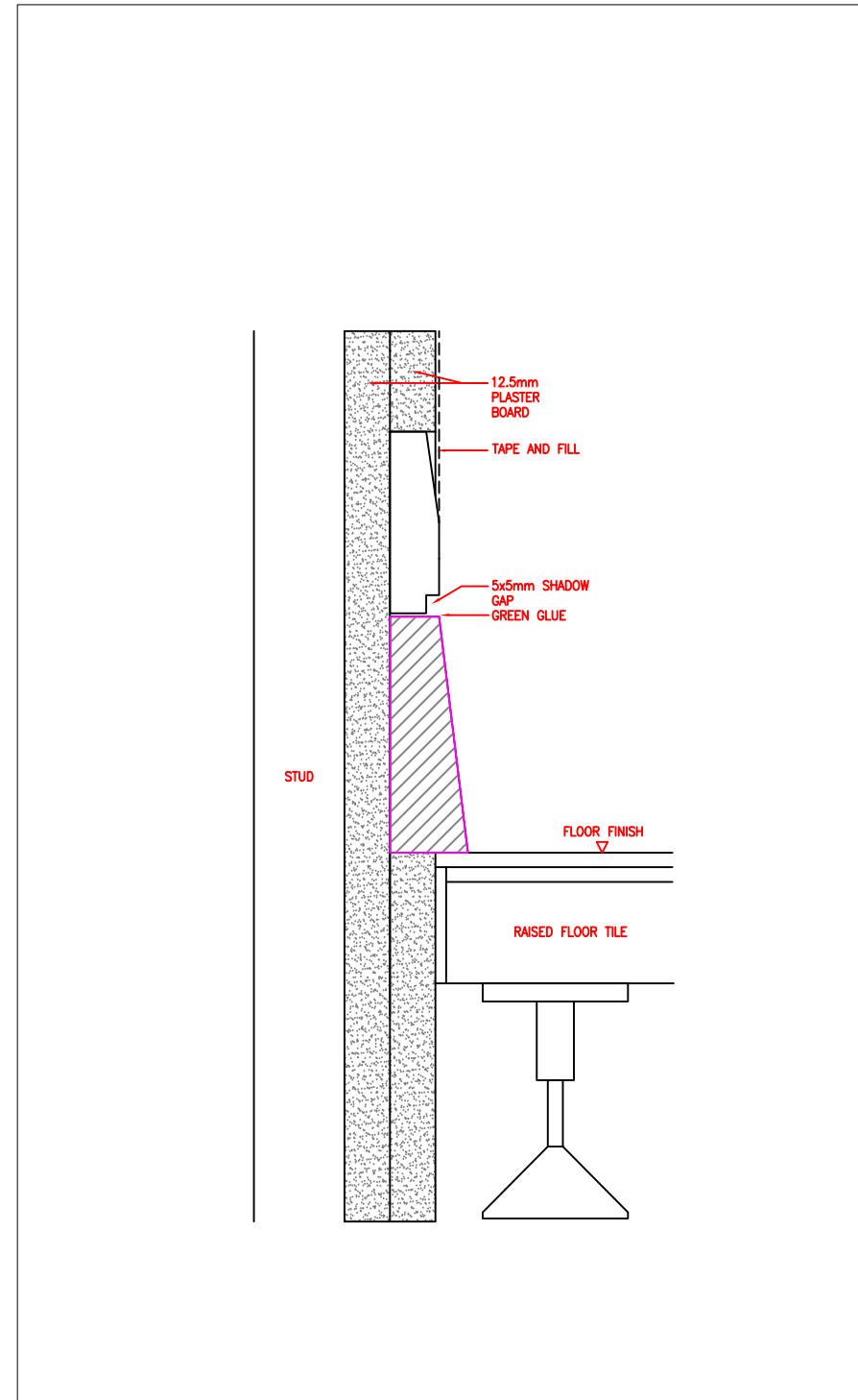
SA ABUTMENT TYPE G 1:2 @ A1
