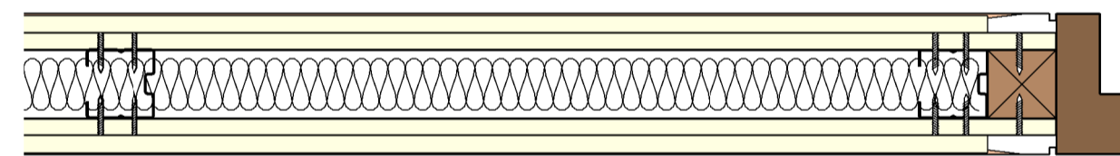
4 Jamb level - SA-16-5- V 1:5
