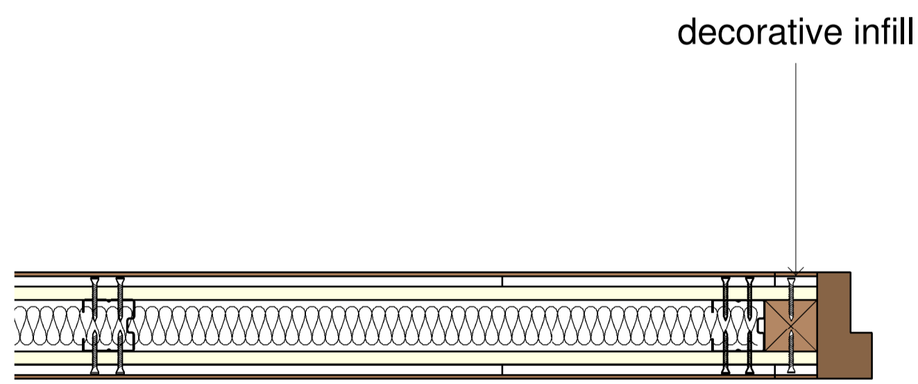
4 Jamb level - SA-16-40-V 1:5
